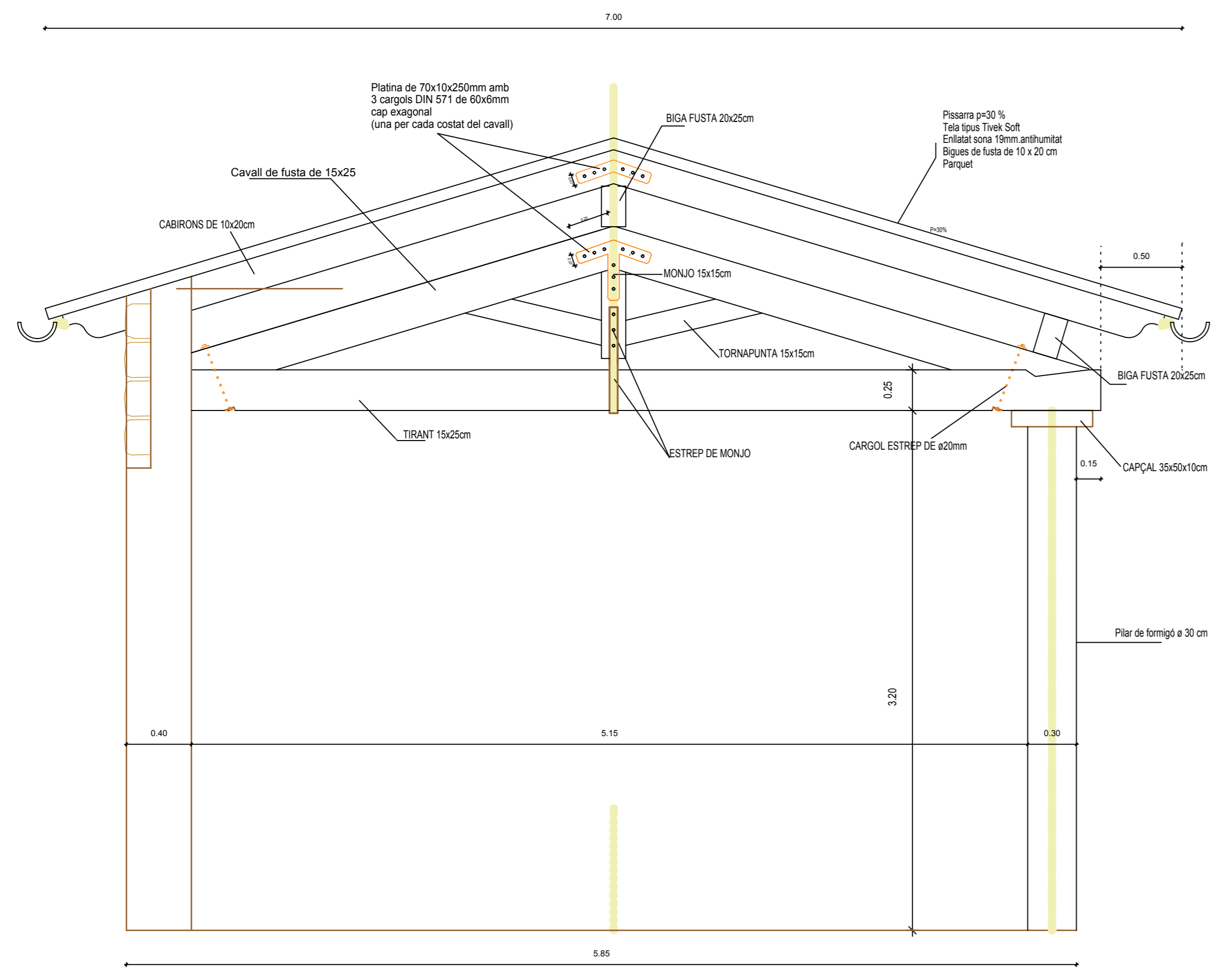
DETALL CAVALL TIPUS DE FUSTA
