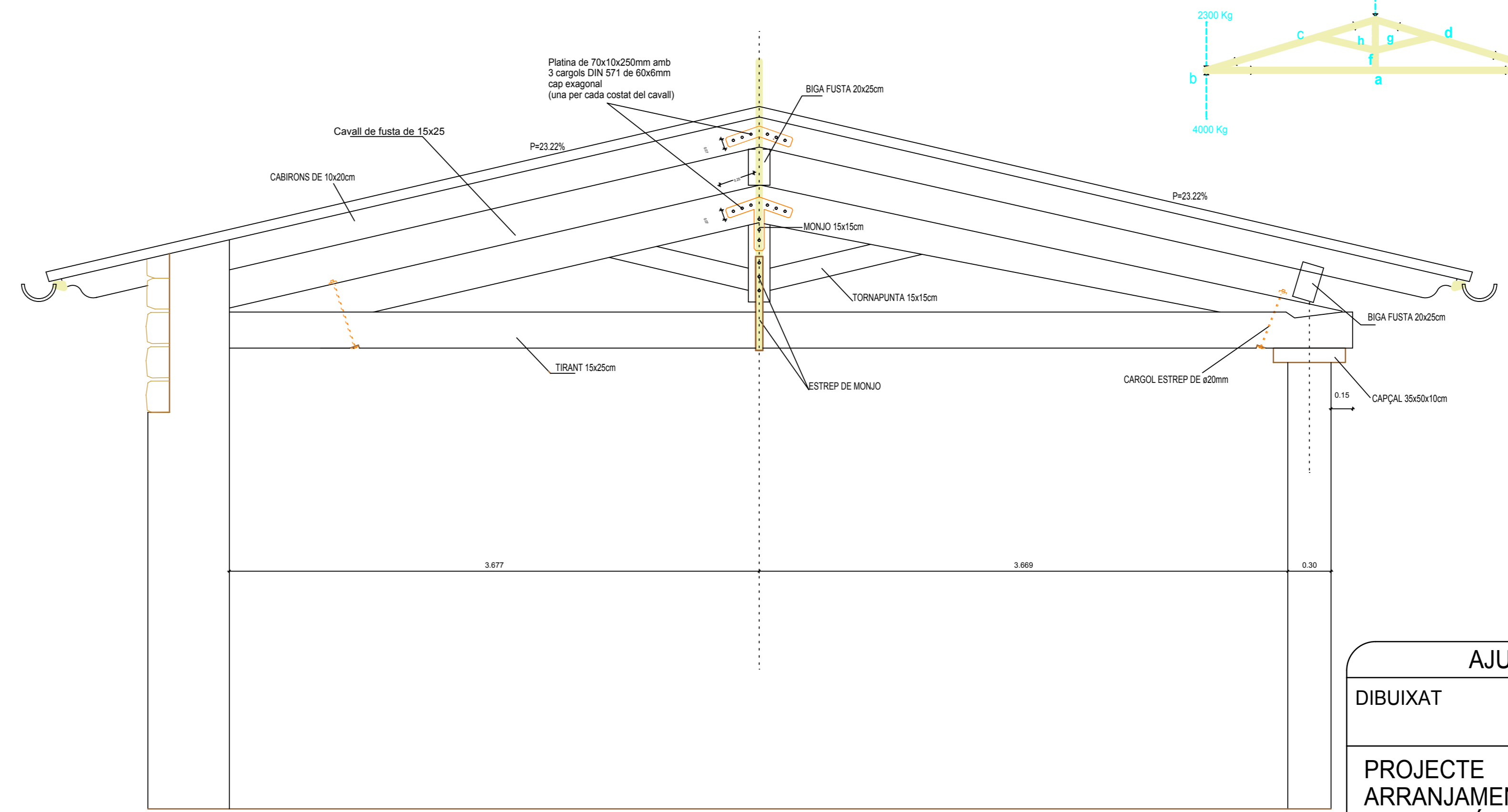
DETALL CAVALL DE FUSTA -INTERSECCIÓ DUES COBERTES-
