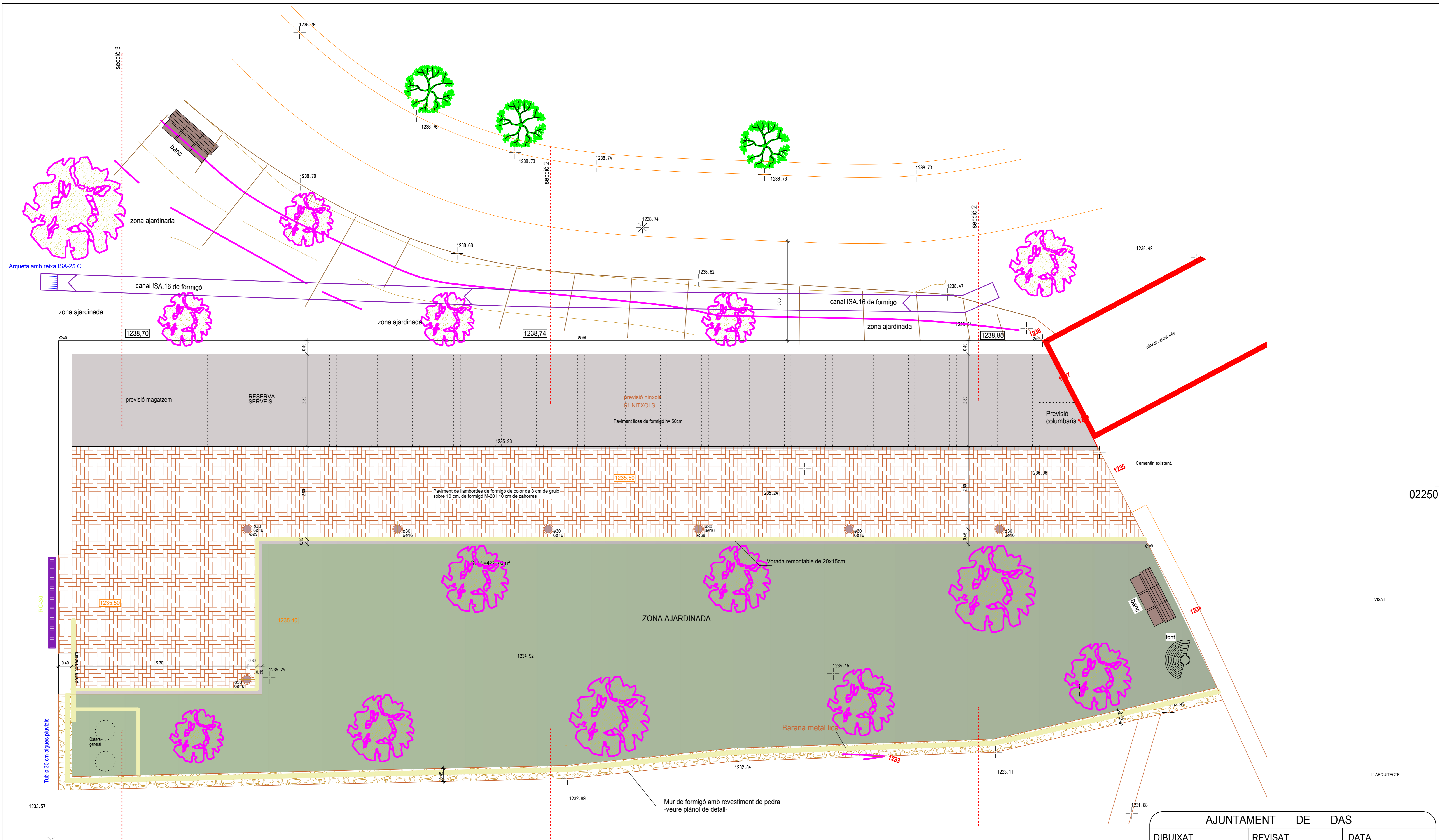
PLANTA CEMENTIRI. SUP.=422,70m 2 ZONA CEMENTIRI TOTAL A AMPLIAR SUP.=2000,00m 2 ----- SECCIONS TRANSVERSALS 1,2,3
