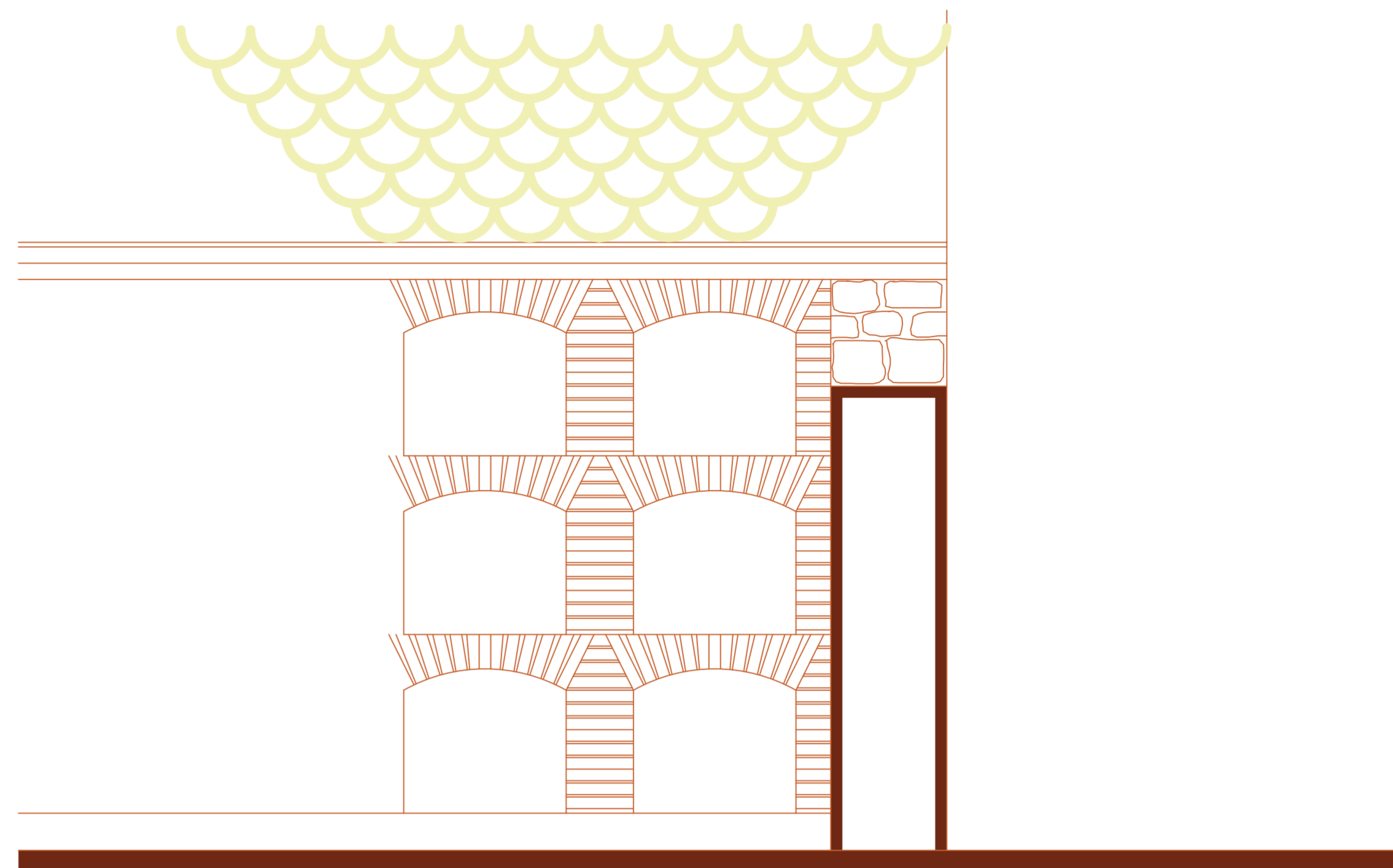
DETALL FAÇANA NINXOLS ESCALA 1 : 20
